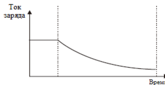
Схема этапов зарядки литиевых аккумулятора (LI)
