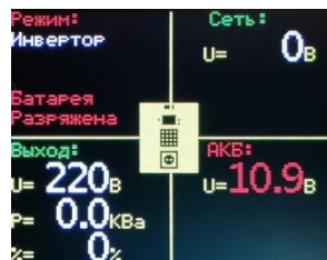
Рис.№4. Индикатор в режиме предупреждения.
