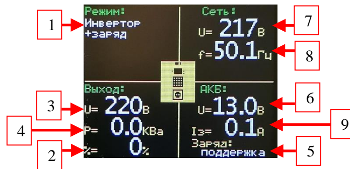
Рис.№2. Индикатор в режиме отображения электрических параметров.
