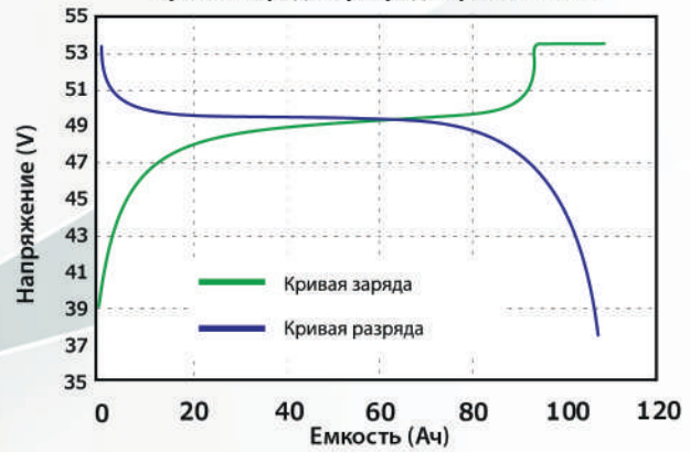
Кривая заряда и разряда при 0.5C 25°C
