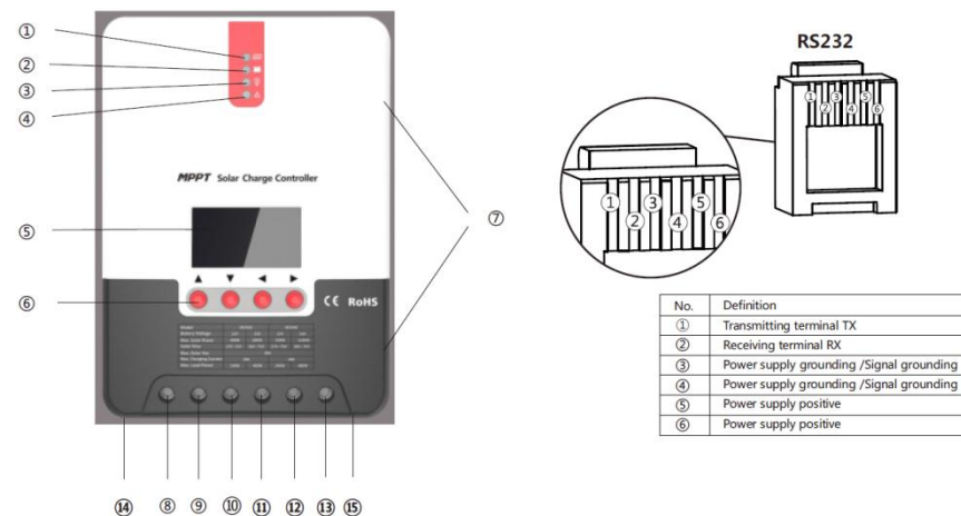
Рисунок 1-1. Внешний вид контроллера и разъемы
