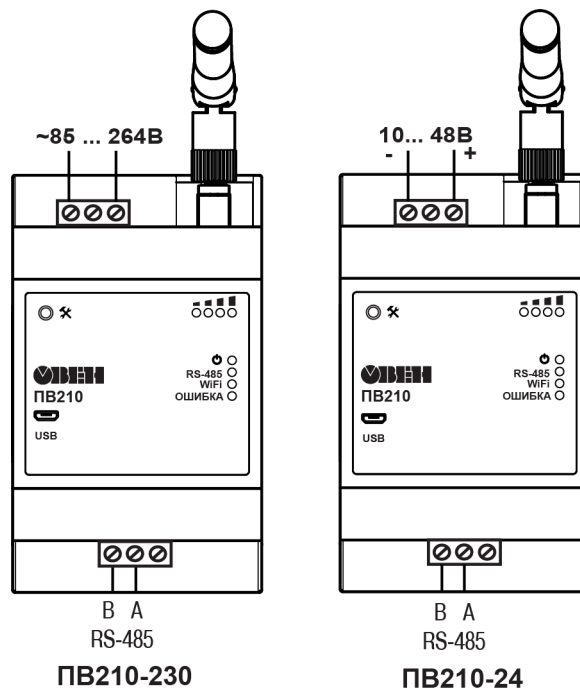
Рисунок 5.1 – Назначение клемм
