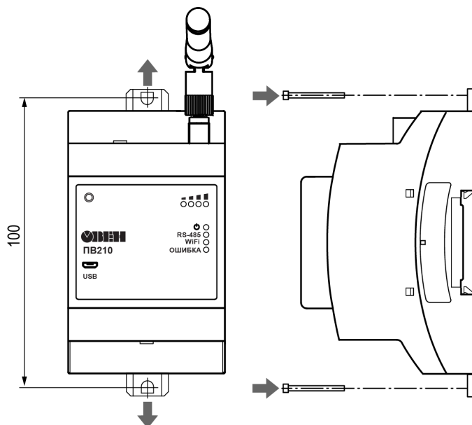
Рисунок 4.2 – Крепление винтами
